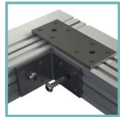
Winkelverstärkung
